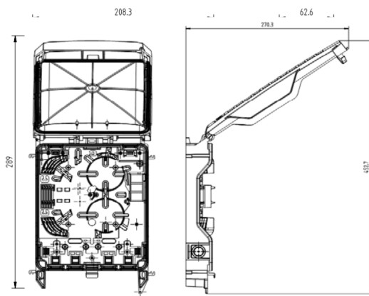
Box mit geöffnetem Deckel
